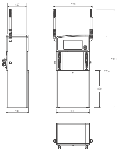
P3000 - 2P2H
